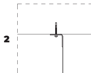
DETALLE DE FIJACIÓN ENTRE ANGULAR Y FORJADO
