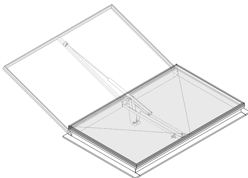
VISTA EN PERSPECTIVA SISTEMA DE APERTURA
