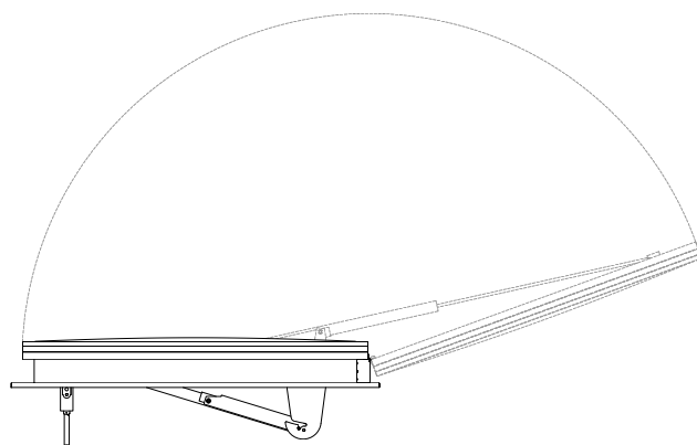
VISTA LATERAL
