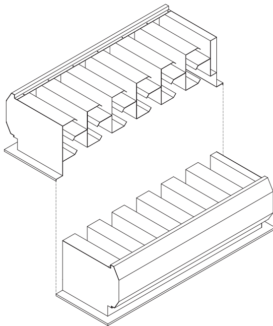
PERSPECTIVA - SECCIÓN S1
