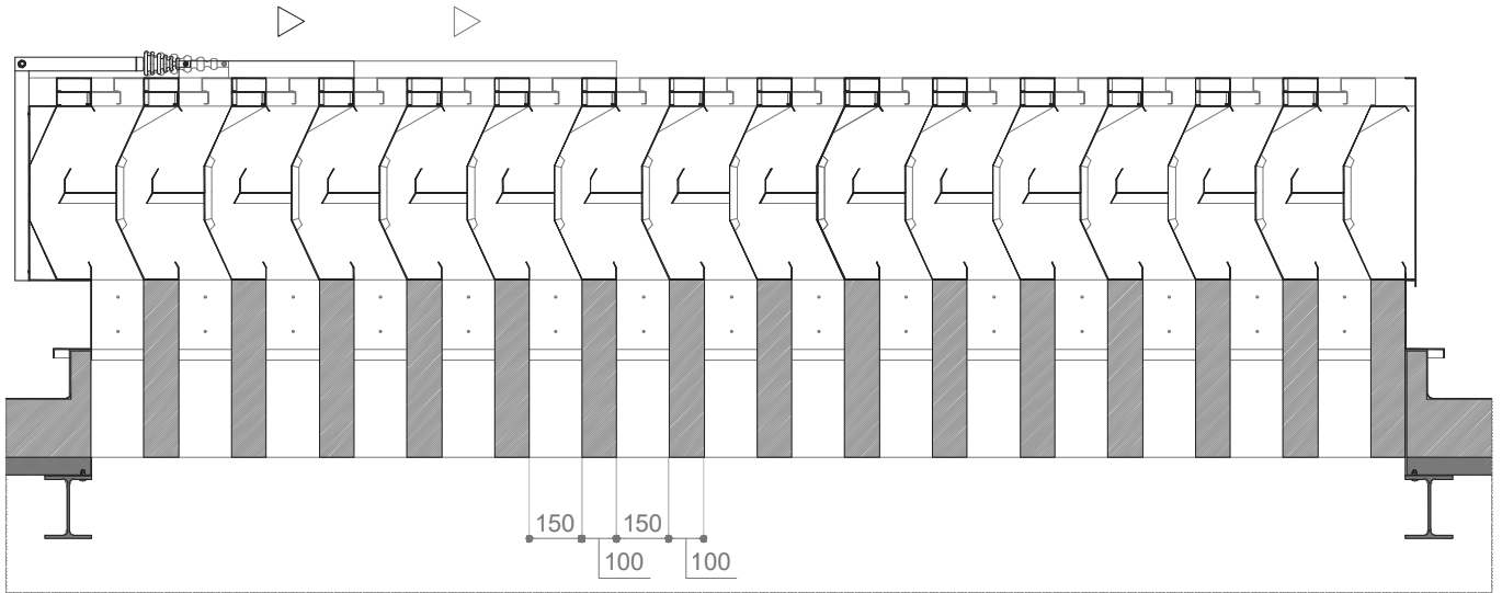
FLUJO DE AIRE 2 CON ATENUADOR DIVISORIO Y DOBLE DESLIZADOR (OPCIONAL).
