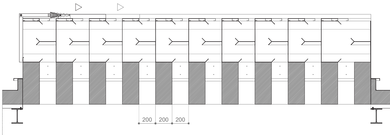
FLUJO DE AIRE 1 CON ATENUADOR DIVISORIO Y MECANISMO DE BLOQUEO (OPCIONAL).
