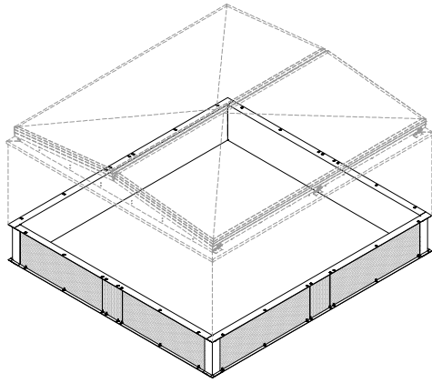
DELTA SHEV ZÓCALO AISLADO VISTA EN PERSPECTIVA
