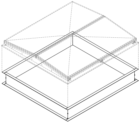
DELTA SHEV ZÓCALO ENSTÁNDAR VISTA EN PERSPECTIVA
